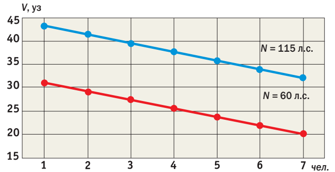
Зависимость скорости от нагрузки при разной мощности
